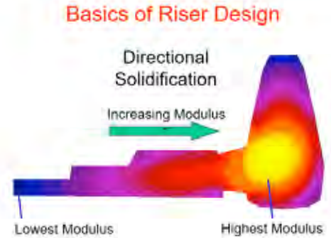
Figura 1. Solidificación Dirigida, desde Módulo bajo hasta Módulo alto.
