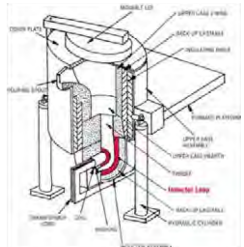
Figura 1. Horno de Inducción a Canal
